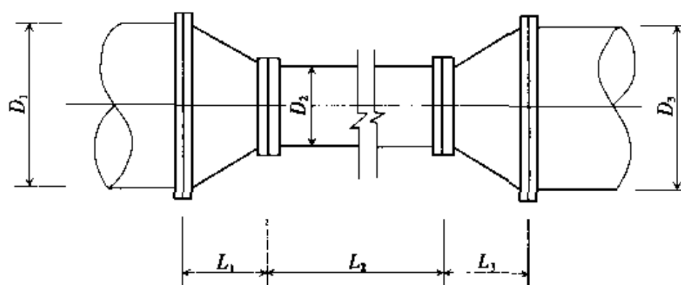
图 22 节流管结构示意图
