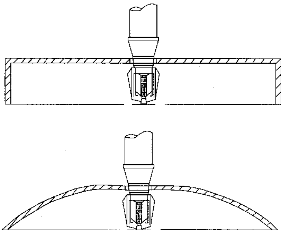
图 14 集热挡水板示意图
