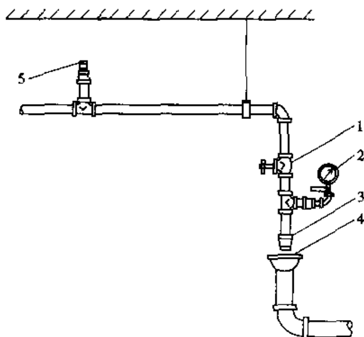
图9 末端试水装置示意图
