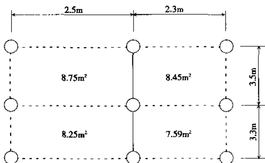
图 20 德国规范中作用面积的举例
