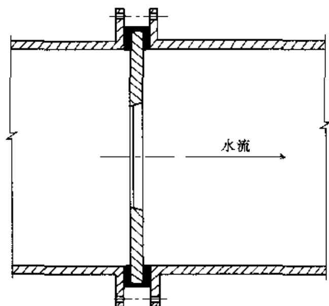
图 21 减压孔板结构示意图
