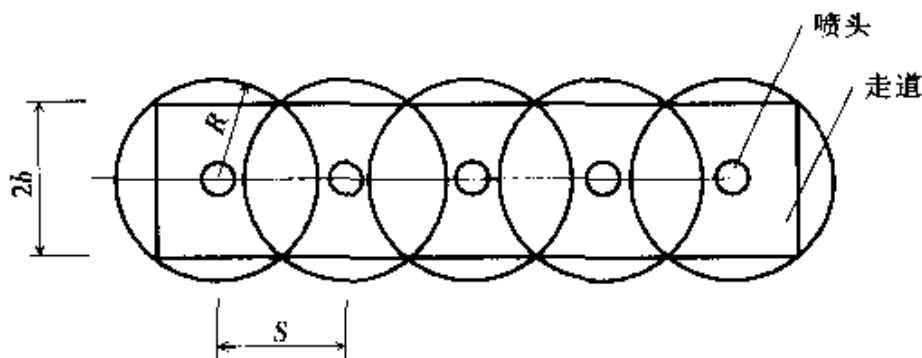
图 8 仅在走廊布置喷头的示意图
