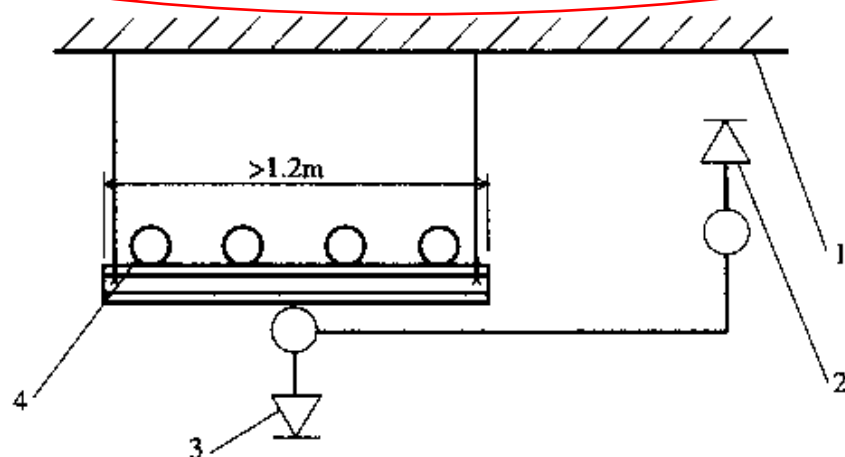
图 7.2.3 障碍物下方增设喷头
