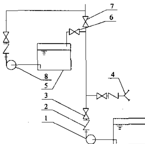
图 25 接力供水设施示意图
