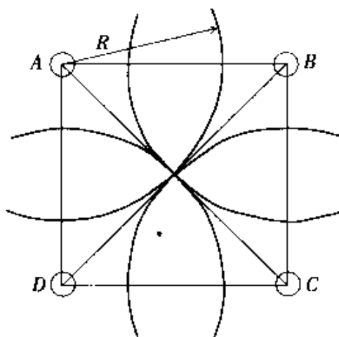
图 10 正方形布置喷头示意图
