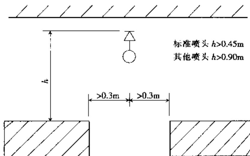
图 13 堆物较高场所通道上方喷头的设置
