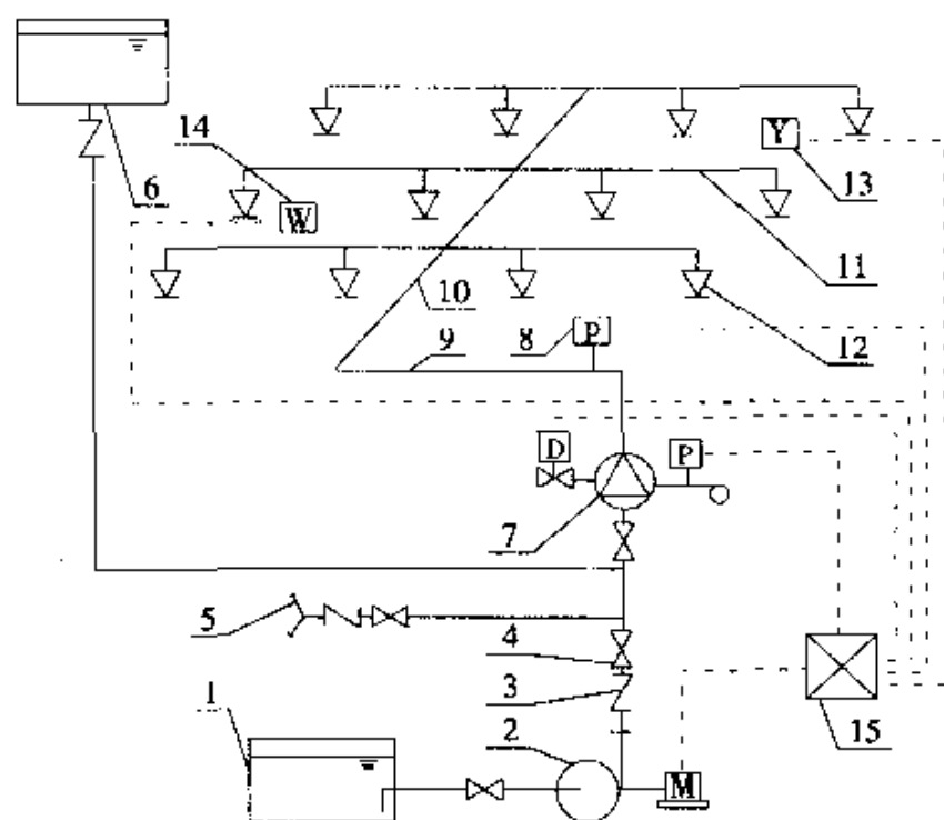
图 4 电动启动雨淋系统示意图
