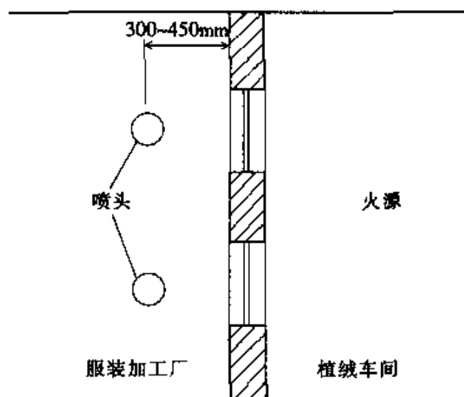
图 15 植绒车间开口外侧设置喷头示意图
