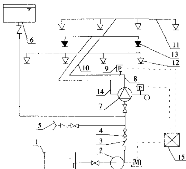
图5 充液(水)传动管启动雨淋系统示意图
