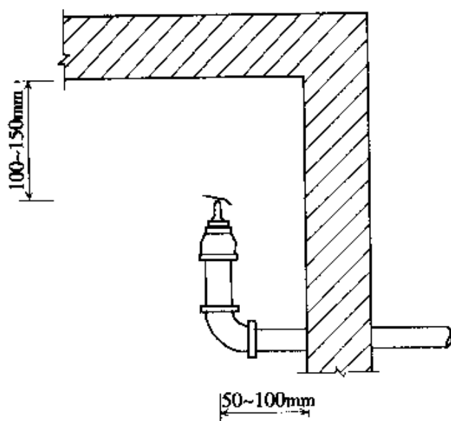
图 18 直立式边墙型喷头的安装示意图
