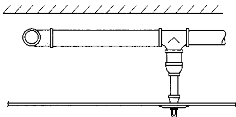
图 12 吊顶下喷头安装示意图
