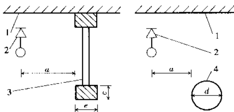
图 7.2.2 喷头与邻近障碍物的最小水平距离
