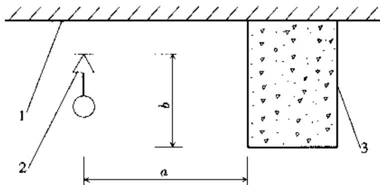
图 7.2.1 喷头与梁、通风管道的距离
