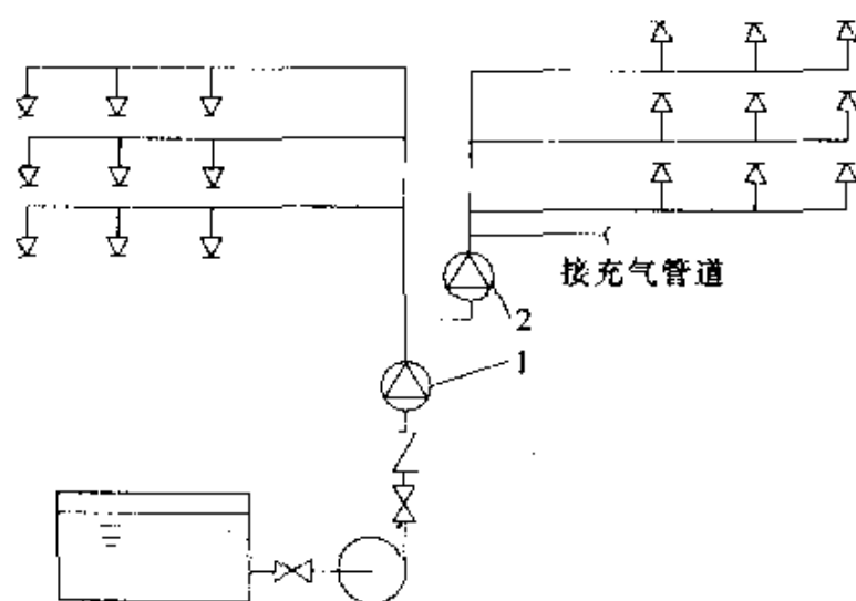
图 6 其他系统接入湿式系统示意图
