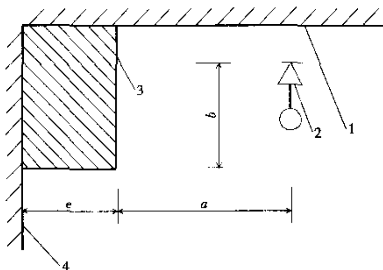
图 7.2.5 喷头与靠墙障碍物的距离
