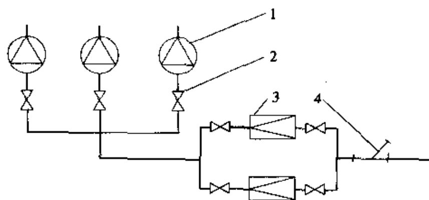
图 23 减压阀安装示意图
