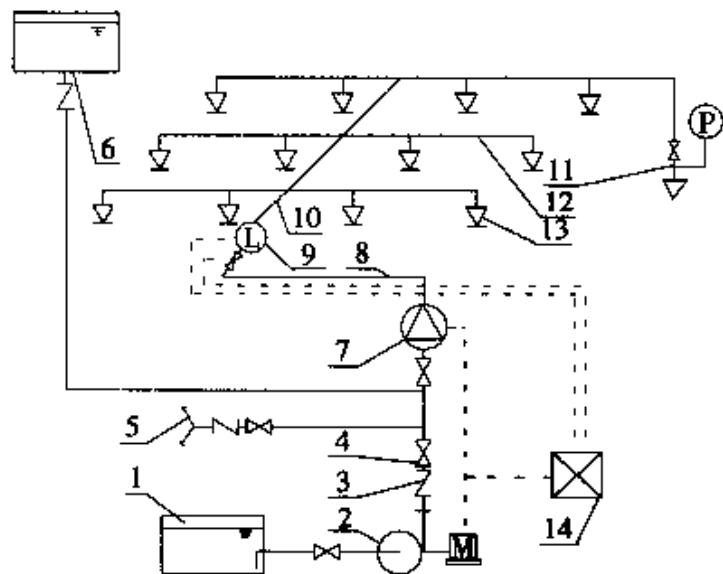
图1 湿式系统示意图
