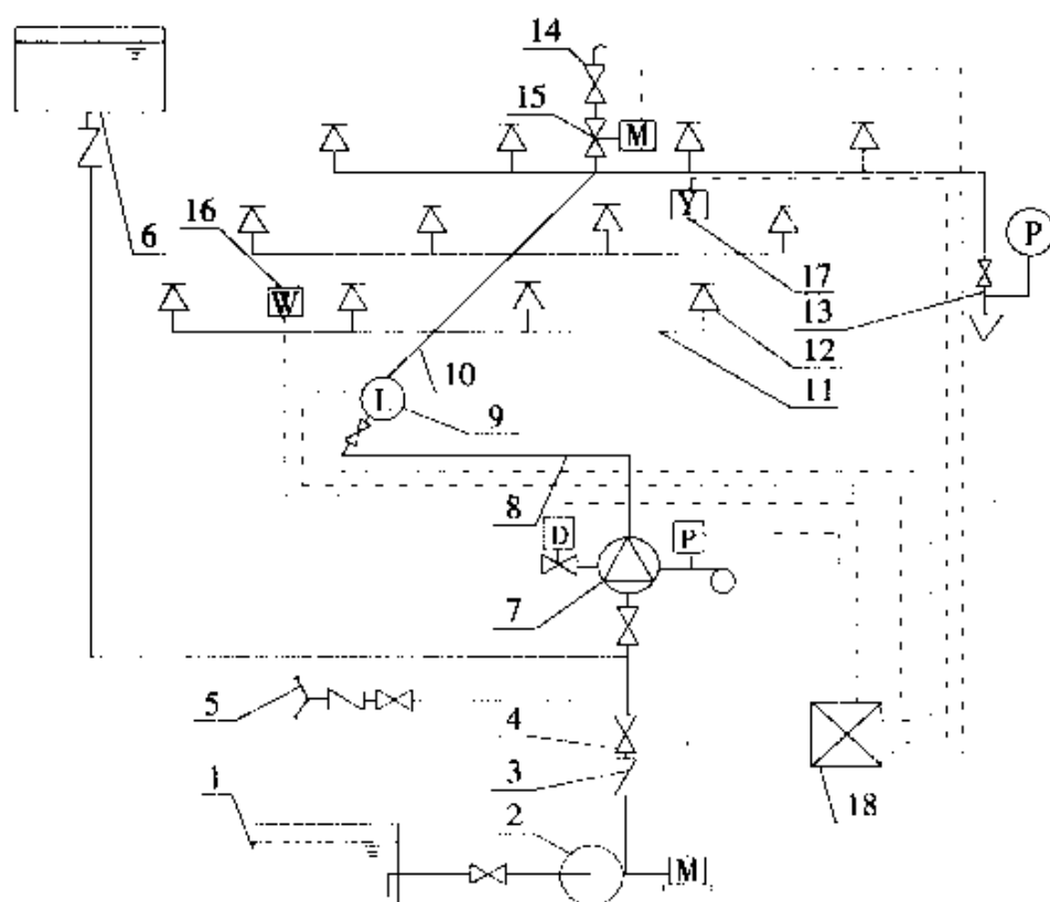
图3 预作用系统示意图
