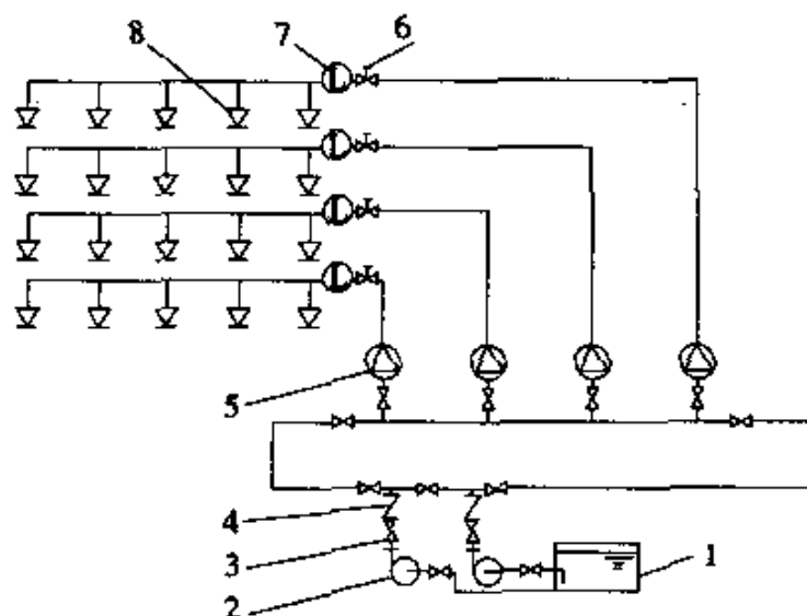
图 24 环状供水示意图
