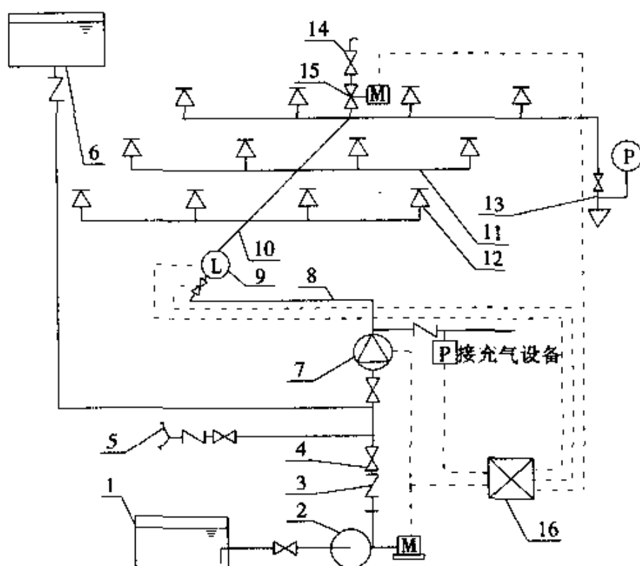
图 2 干式系统示意图
