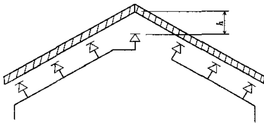
图 16 屋脊处设置喷头示意图
