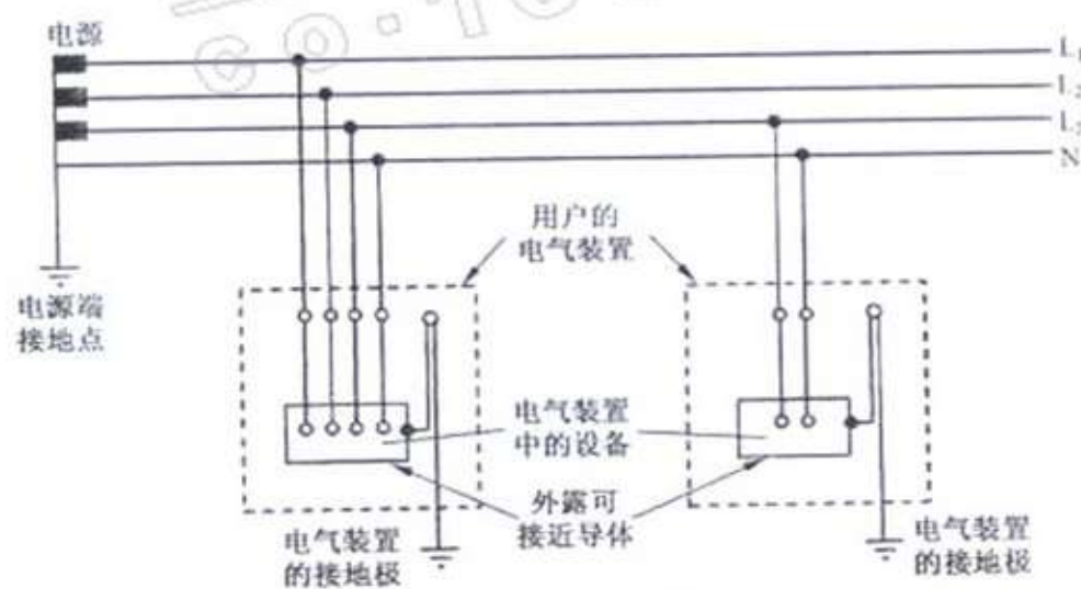
图 A.4 TT 系统
