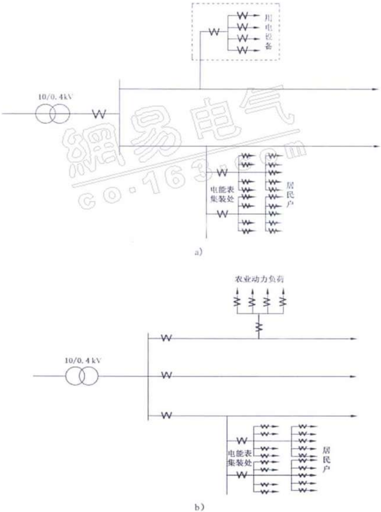
图 C.1 分级保护方式参考模式图
