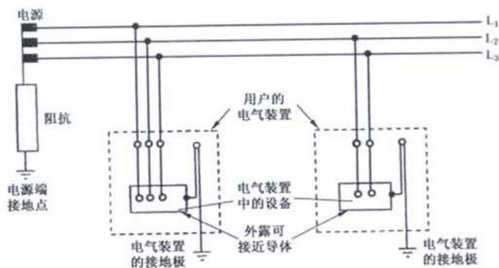
图 A.5 IT 系统
