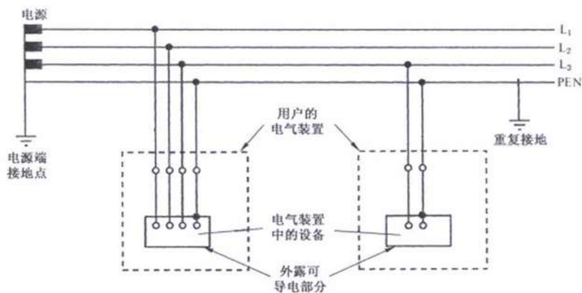
图 A.2 TN-C 系统
