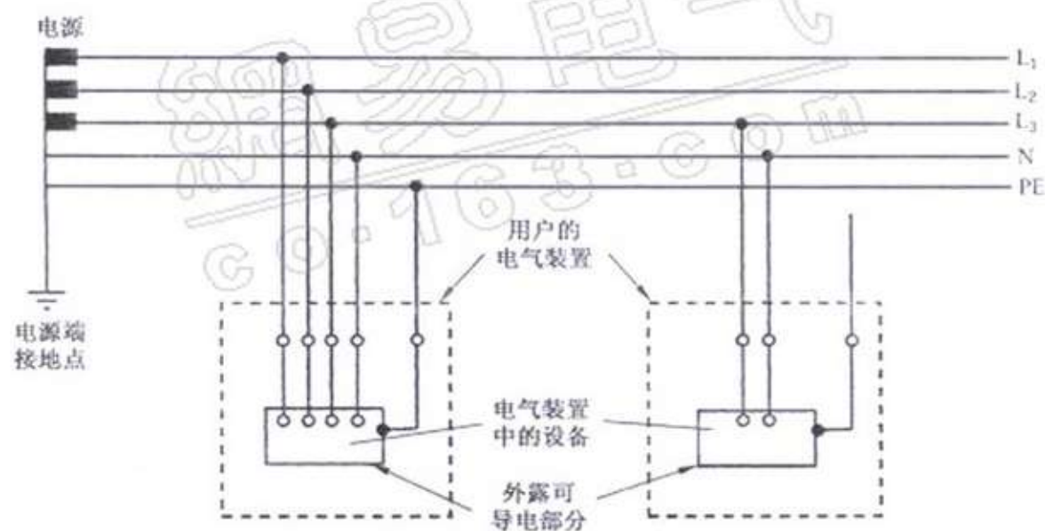
图 A.1 TN-S 系统
