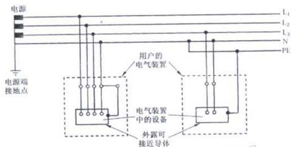
图 A.3 TN-C-S 系统
