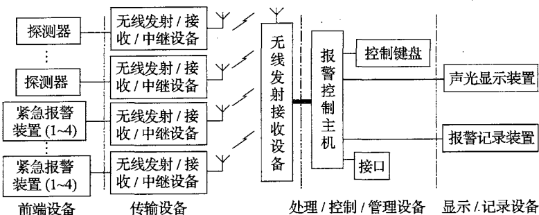
图 4.0.2-3 无线制模式
