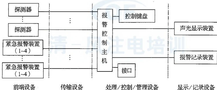
图 4.0.2-1 分线制模式
