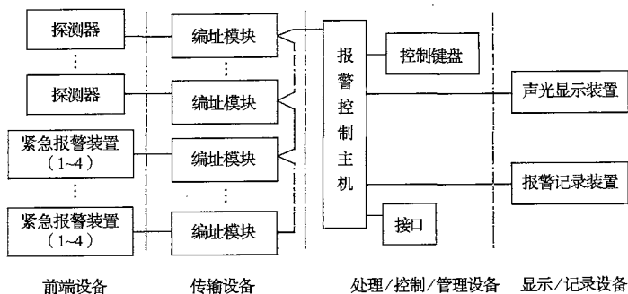
图 4.0.2-2 总线制模式
