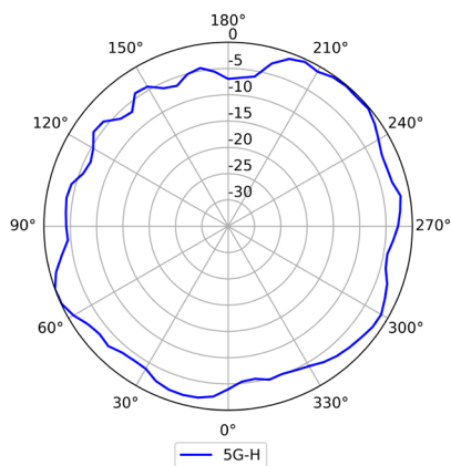
5GHz (水平)
