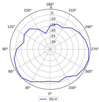
5GHz (垂直)
