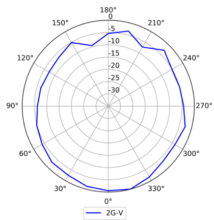
2.4GHz (垂直)
