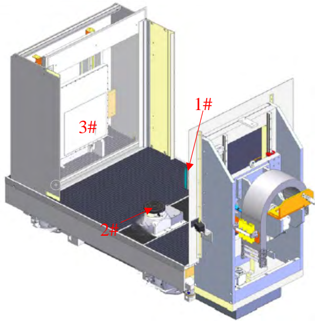
图 9-4 设备内部结构图
