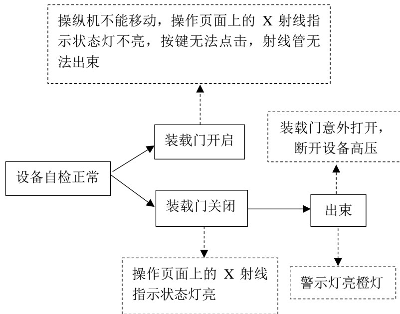
图 10-6 门机联锁逻辑图
