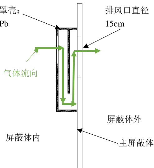
图 10-4 排风口屏蔽补偿示意图
