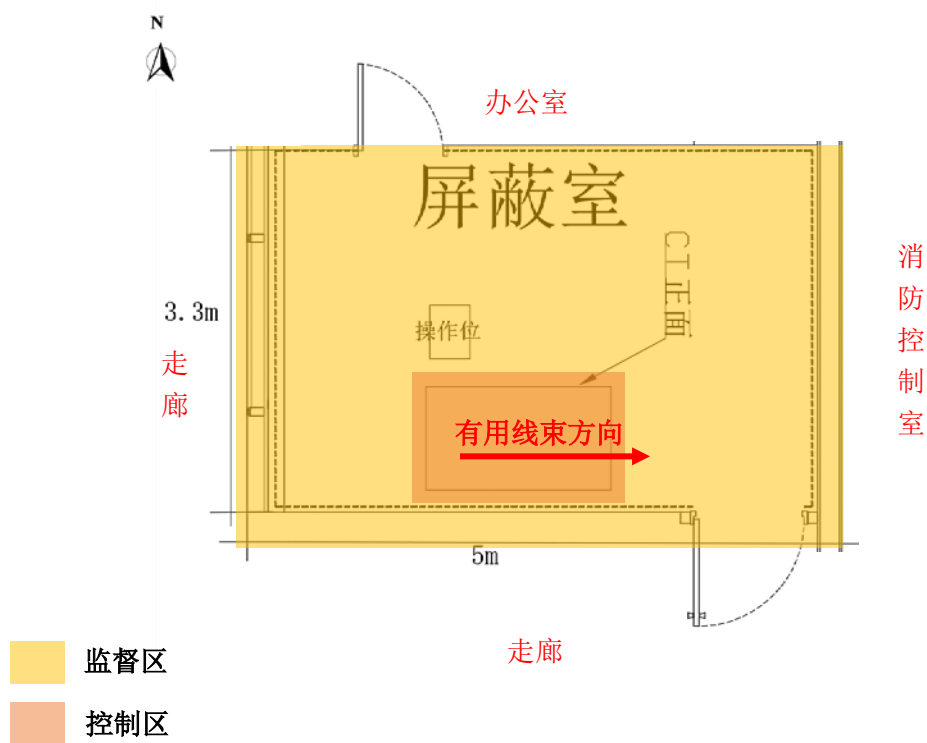
图 10-8 辐射工作场所布局和分区示意图
