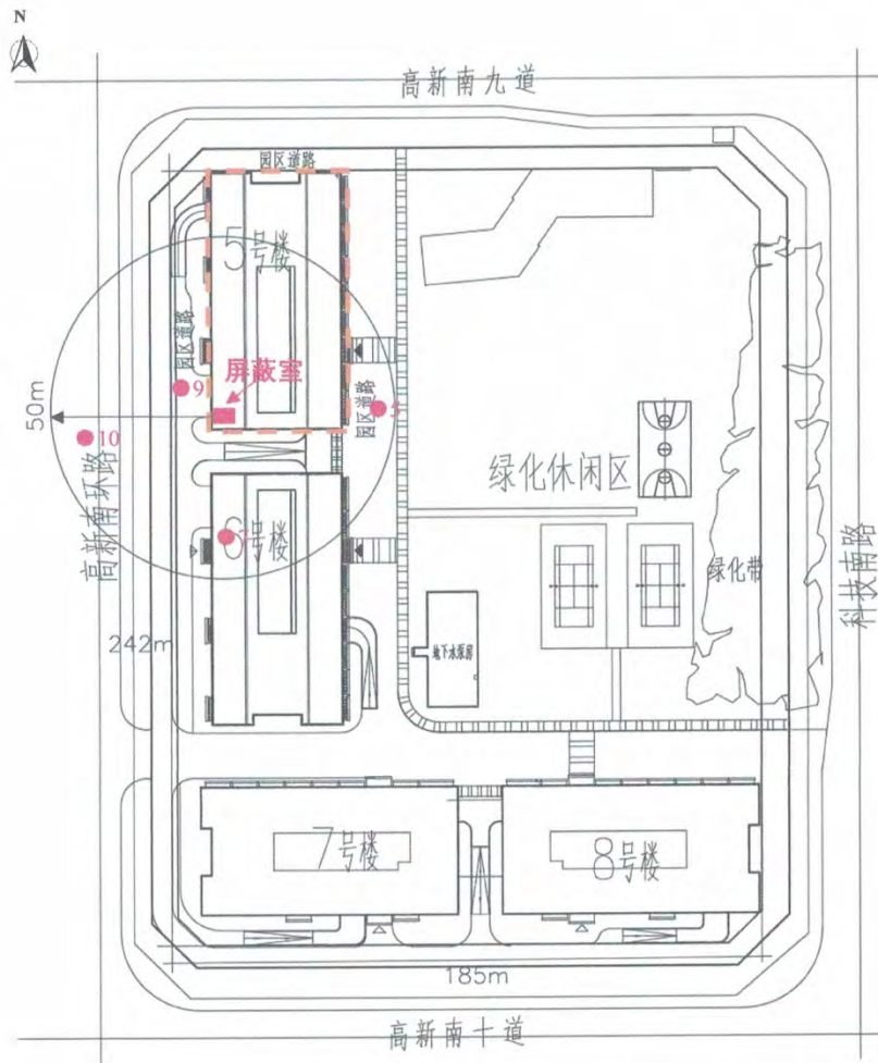
50m 评价范围内检测布点图
