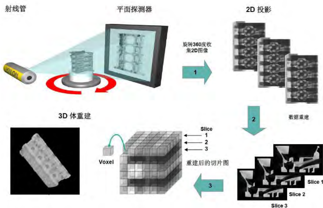
图 9-2 工业 CT 工作原理示意图
