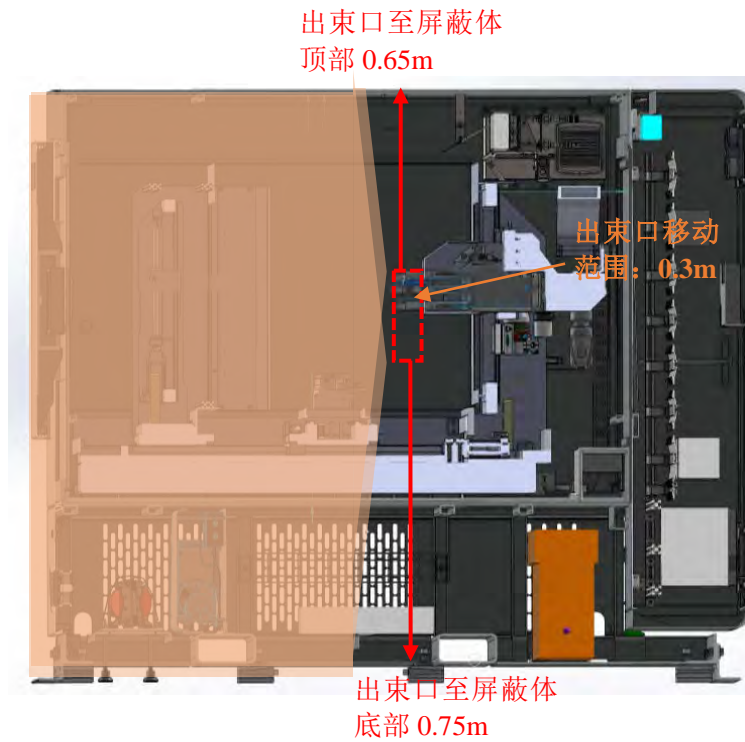
图 11-1 射线管分布示意图
