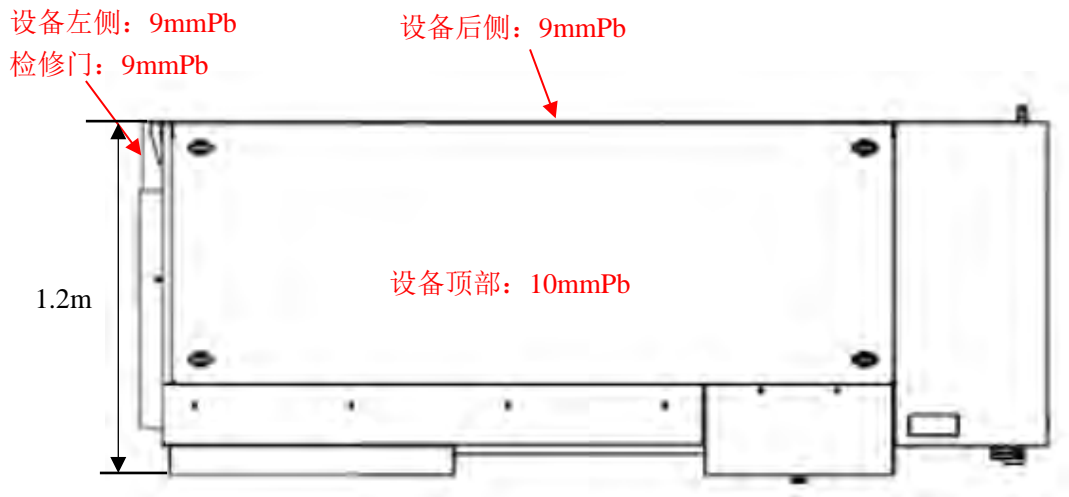
图 10-2 射线装置俯视图
