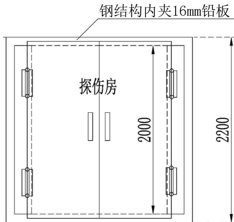
图 10-2 探伤房立面设计图 (单位: mm)
