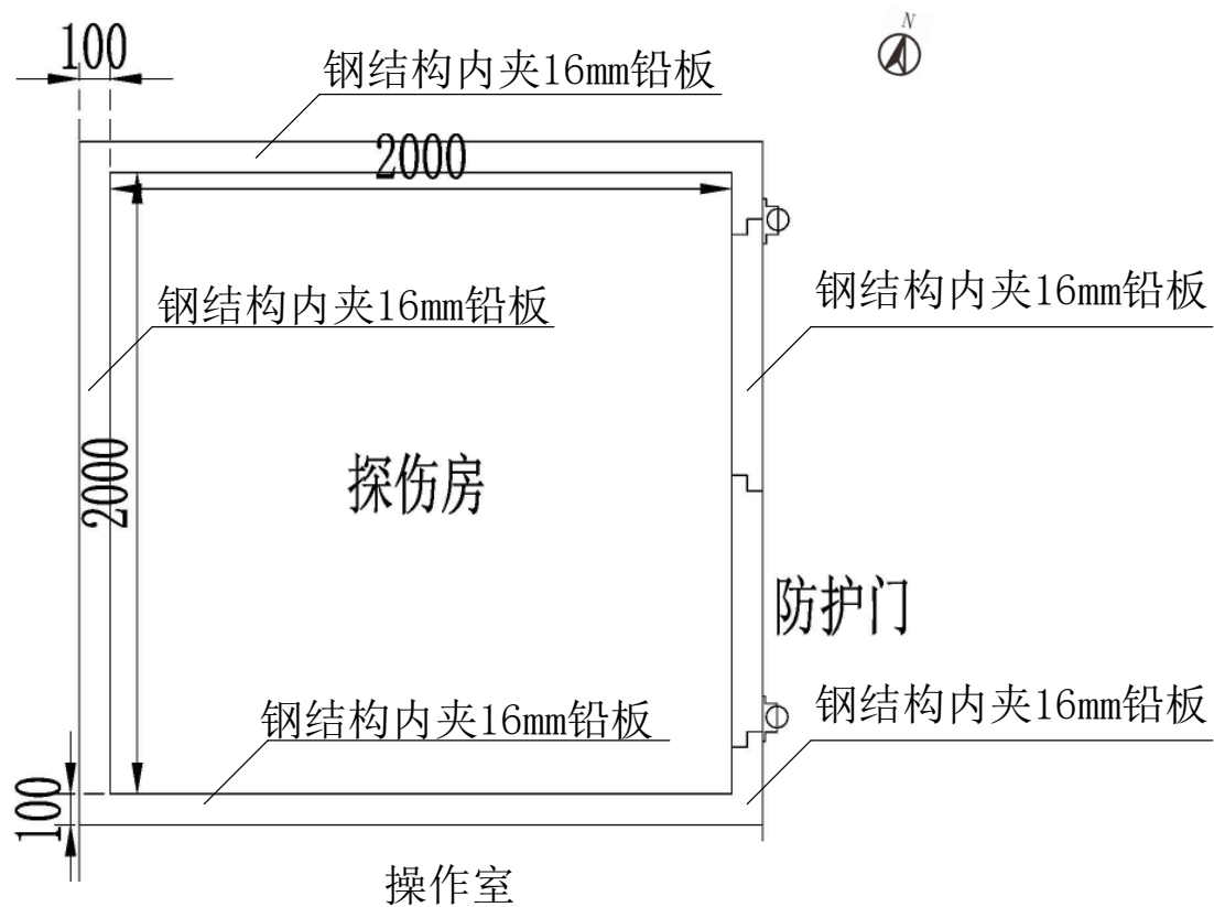
图 10-1 探伤房平面设计图 (单位: mm)
