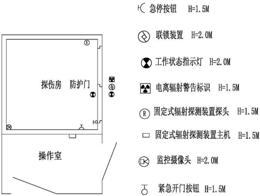
图 10-8 辐射安全与防护设施分布图
