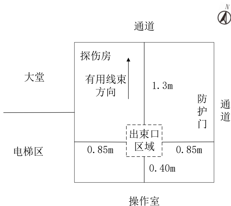
图 11-1 出束口区域示意图（平面）
