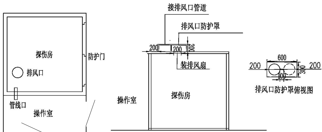
图 10-5 排风口位置和防护罩设计示意图（单位：mm）
