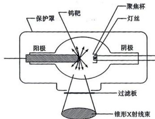
图 9-2 X 射线产生的示意图
