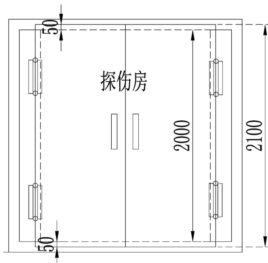
图 10-4 防护门上下搭接示意图（单位：mm）
