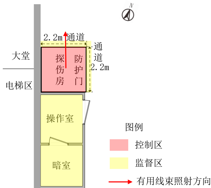
图 10-9 辐射工作场所布局和分区示意图
