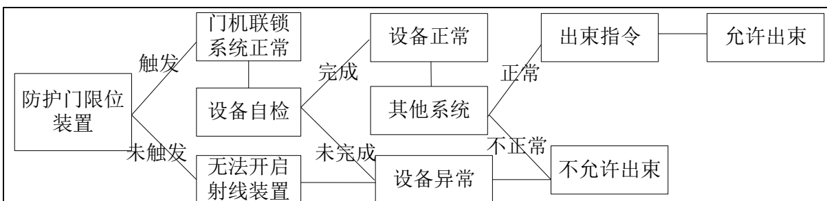
图 10-7 门机联锁逻辑图
