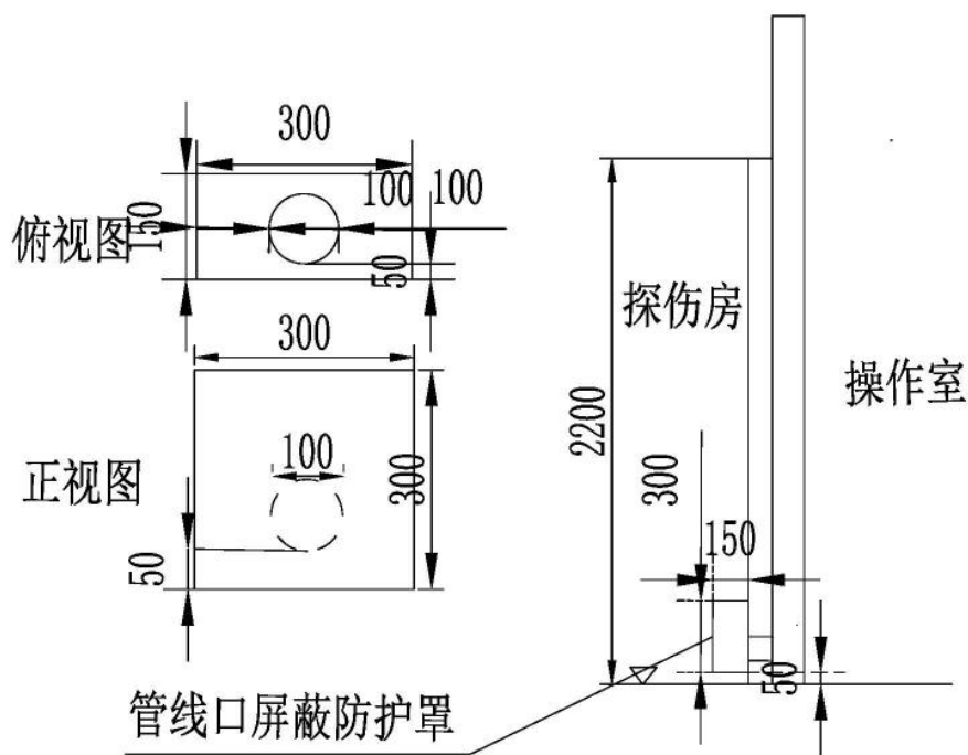
图 10-6 管线口防护罩设计示意图（单位：mm）
