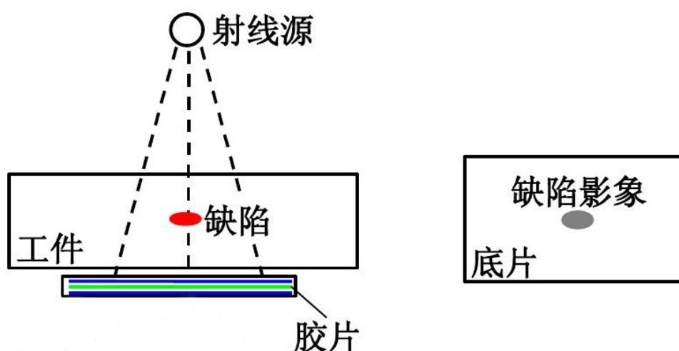
图 9-3 X 射线胶片成像示意图
